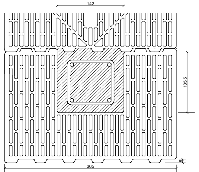
Réalisation d'un poteau en 365 mm
