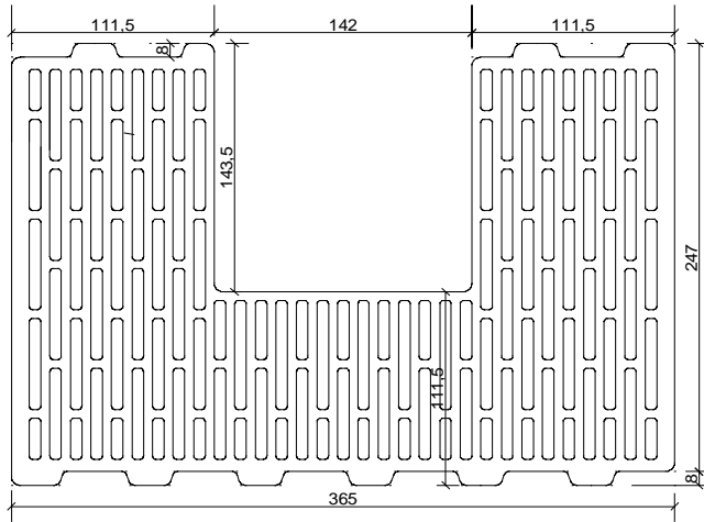
Brique 3B Poteau en 365 mm
